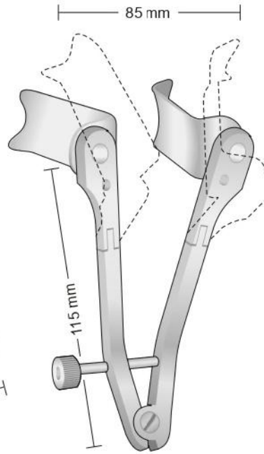
CASPAR SSQ-9399-1 Completo con 5 valve Complete with 5 blade Komplett mit 5 Blätter Complet : 5 valves Completc 5 valvas
