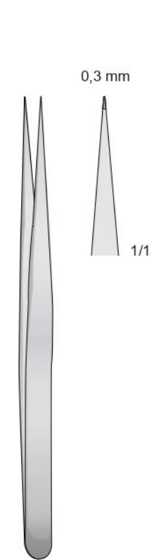
SSQ-10701-1 120 mm
